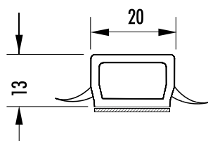
GL 2013-S-L Schaumklebeband schwarz
