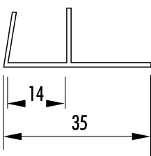
UW 35 | Wandstärke 1,0 mm
