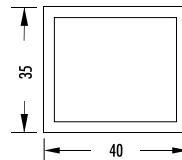
R 4035 | Wandstärke 3,0 mm
