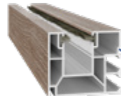
Rolladen- führungsschiene 40 x 47 mm Dekor auf den Sichtseiten
