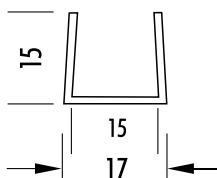
U 15 15 15 | Wandstärke 1,0 mm
