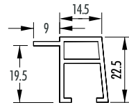
KA 2720 (passend: NI 935)
