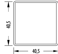
R 4040 | Wandstärke 1,4 mm
