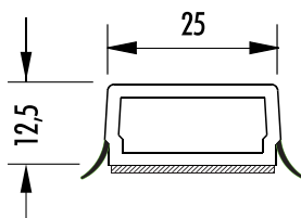
GL 25125-S-L Schaumklebeband schwarz
