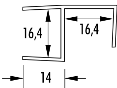
V 16 | Wandstärke 1,2 mm
