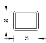
R 2520 | Wandstärke 2,0 mm
