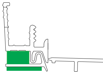
DS8776 Anputzdichtleiste-Rain Außen
