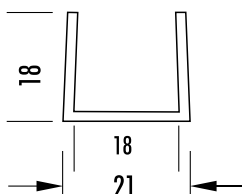
U 18 18 18 | Wandstärke 1,5 mm
