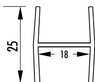
H 1825 | Wandstärke 1,2 mm
