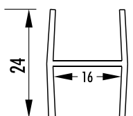
H 1624 | Wandstärke 1,2 mm
