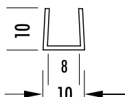
U 10 8 10 | Wandstärke 1,0 mm
