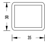
R 3530 | Wandstärke 3,0 mm
