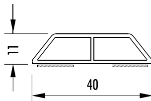
GL 4011-S Schaumklebeband 2 x 12 mm weiß
