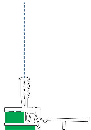
DS8786 Anputzdichtleiste WDVS Außen
