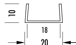
U 10 18 10 | Wandstärke 1,0 mm
