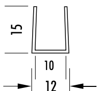
U 15 10 15 | Wandstärke 1,0 mm
