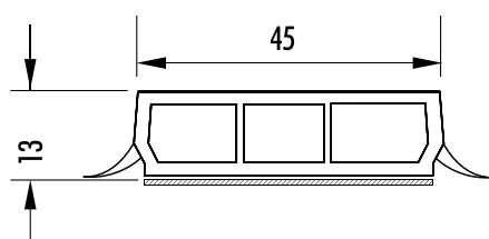
GL 4513-S-L Schaumklebeband schwarz
