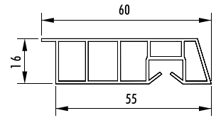
KA 6016 (passend: NI 410)
