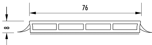
GL 7608-S-L Schaumklebeband schwarz
