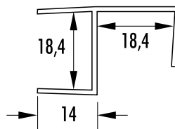
V 18 | Wandstärke 1,2 mm
