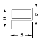
R 2815 | Wandstärke 2,0 mm
