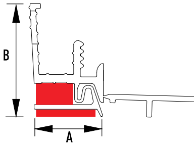
DS8766 Anputzdichtleiste-Air Membran Innen
