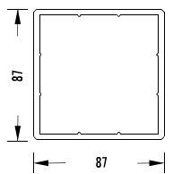
SP8787 | Pfostenprofil 87 x 87 mm
