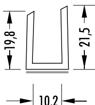
UW 10-S | Wandstärke 2,5 mm dünnnes Klebeband 12,0 mm
