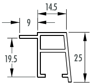
DL 2723 | Wandstärke 1,5 mm
