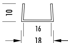
U 10 16 10 | Wandstärke 1,0 mm
