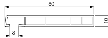
KP80 (passend: NI 951)
