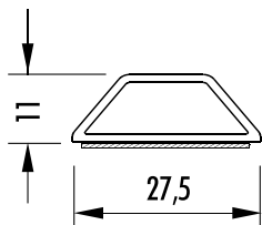
GL 2811-S Schaumklebeband 25 mm weiß
