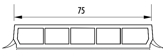
GL 25125-S-L Schaumklebeband schwarz
